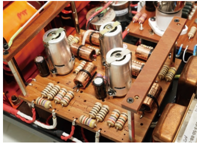
E. M8 Phono MM唱放部分採用多重獨立屏蔽，以三支JAN 5670W作兩級放大，並大量採用Audio Note名貴純銀的薄膜非磁性電容器及Tantalum鉭膜非磁性電阻器，全銀兼手工搭棚式接駁電路製作，全採用經處理的實木夾板充當電路基板
