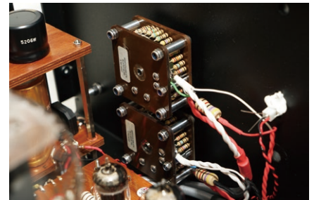
L. Audio Note自家製獨立Tantalum鉭膜電阻砌成的36級級進式音量調節器
