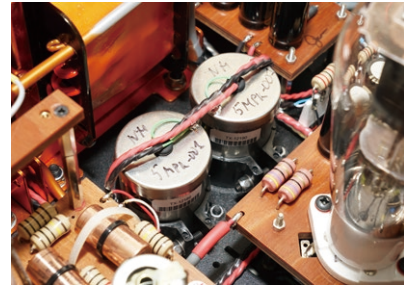
F. 自家製XLR平衡輸入變壓器（純銀線繞輸入/輸出級），左、右兩聲道的各藏在兩個金屬屏蔽殼之內
