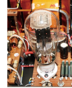
I. 功率放大級真空管4300E（Audio Note專有300B膽型號）
